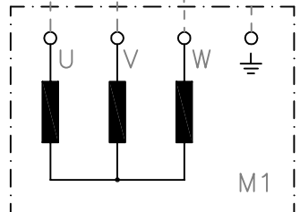
Sternverschaltung
