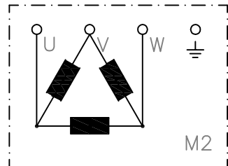
Dreieckverschaltung
