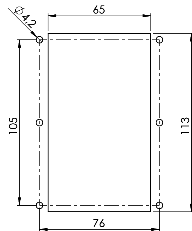
Einbaumaße
