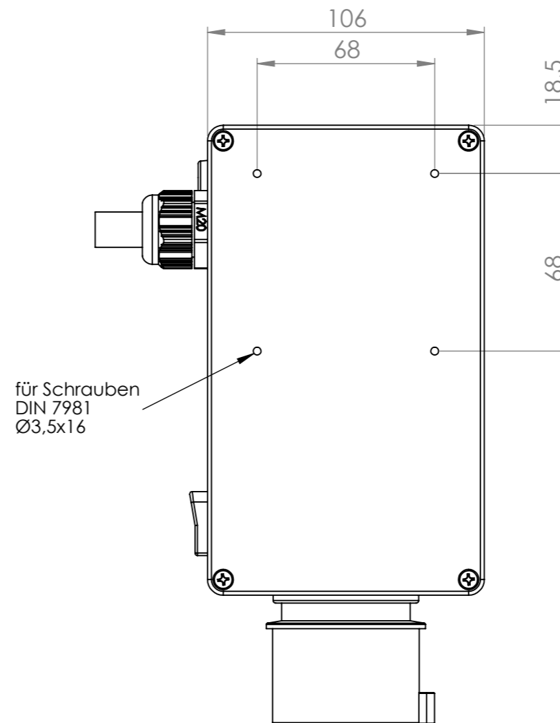
Ansicht "A"
