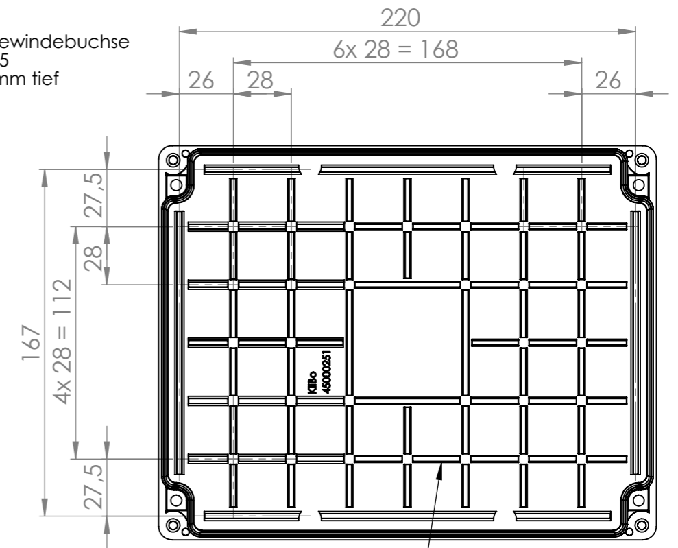
Innenansicht Unterteil
