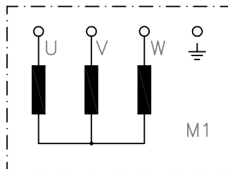
Sternverschlaltung
