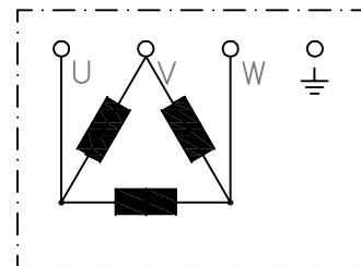
Dreieckverschlaltung
