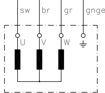
Sternverschaltung
